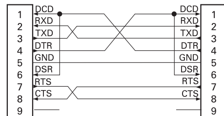
DB-9S-Steckverbinder für Datenübertragungseinrichtung
