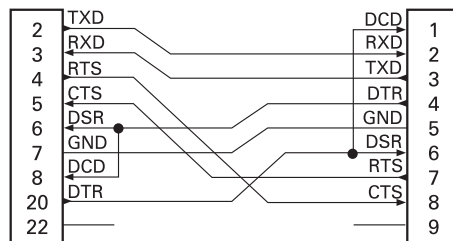
DB-25S-Steckverbinder für Datenübertragungseinrichtung
